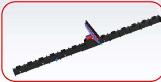
OCP12V汇流母排（与横母排通过螺钉连接实现功率输入架构）
